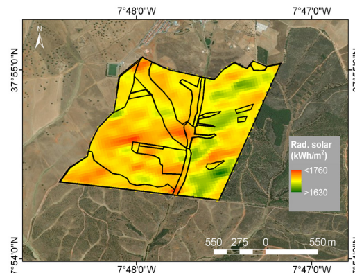
Figura 4 - Mapa da radiação global média anual.
