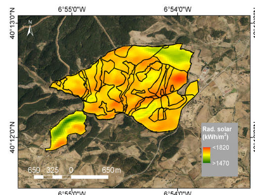
Figura 4 - Mapa de irradiación solar global media anual.
