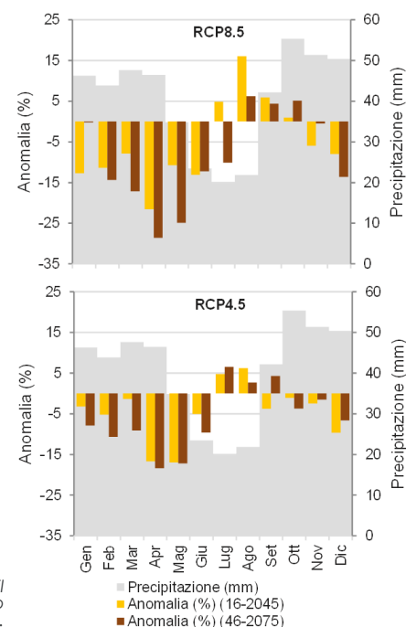
Figura 6 – Precipitazioni medie mensili per il periodo storico; anomalie nel breve e lungo termine, per gli scenari RCP4.5 e 8.5.
