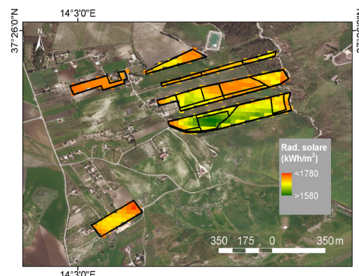
Figura 4 – Mappa della radiazione solare media annua.
